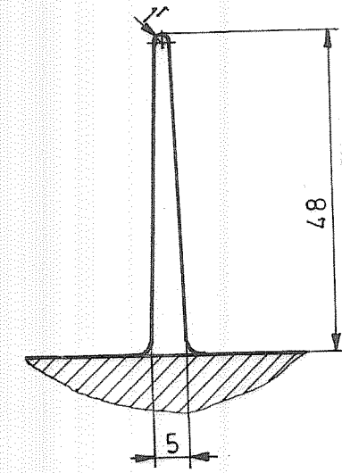
F-F KISMI KESİTİ
