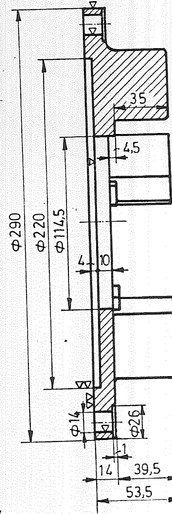
A-A KESİTİ
