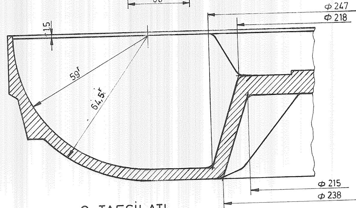
C-TAFSİLATI
