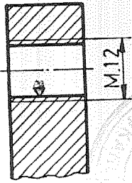
B-B KESİTİ
