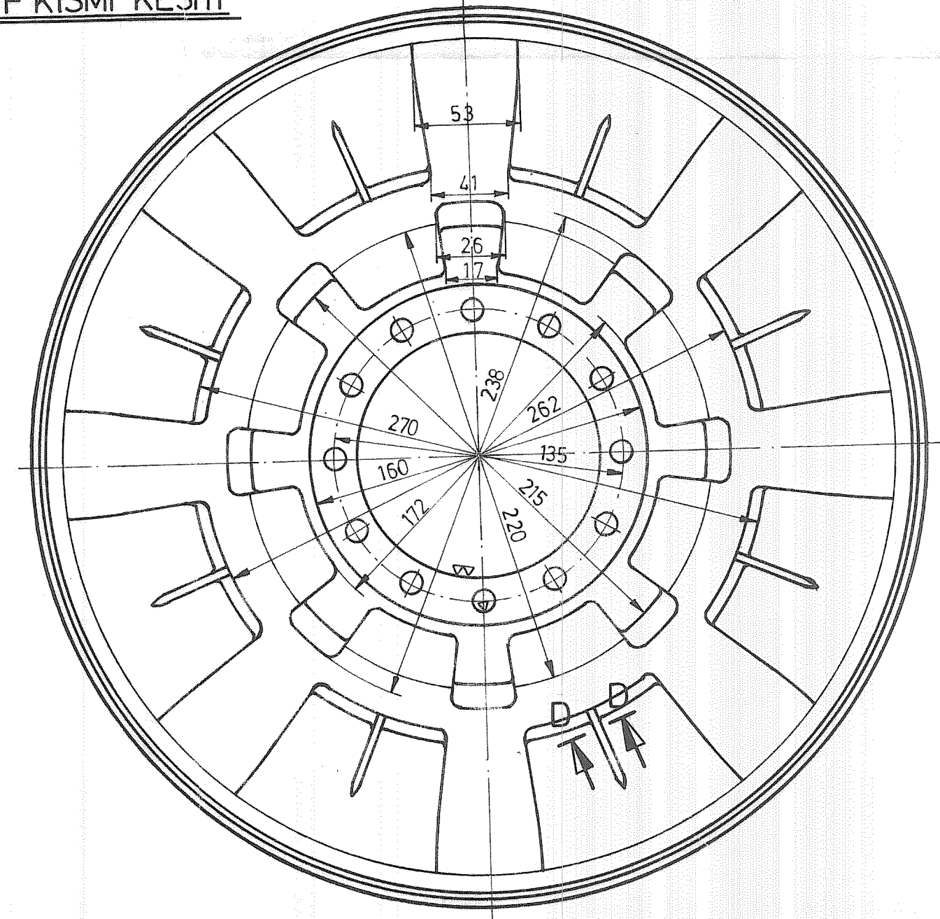
F-F KISMI KESİTİ
