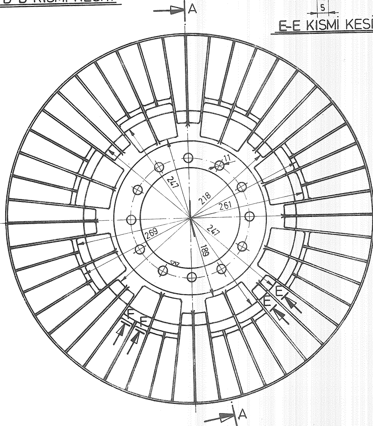
D-D KISMI KESİTİ
